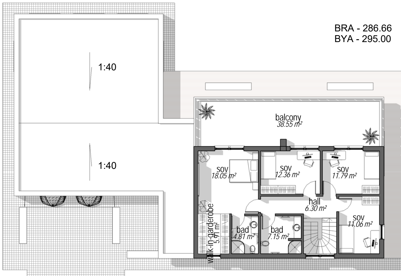
1 floor plan M 1 : 150
