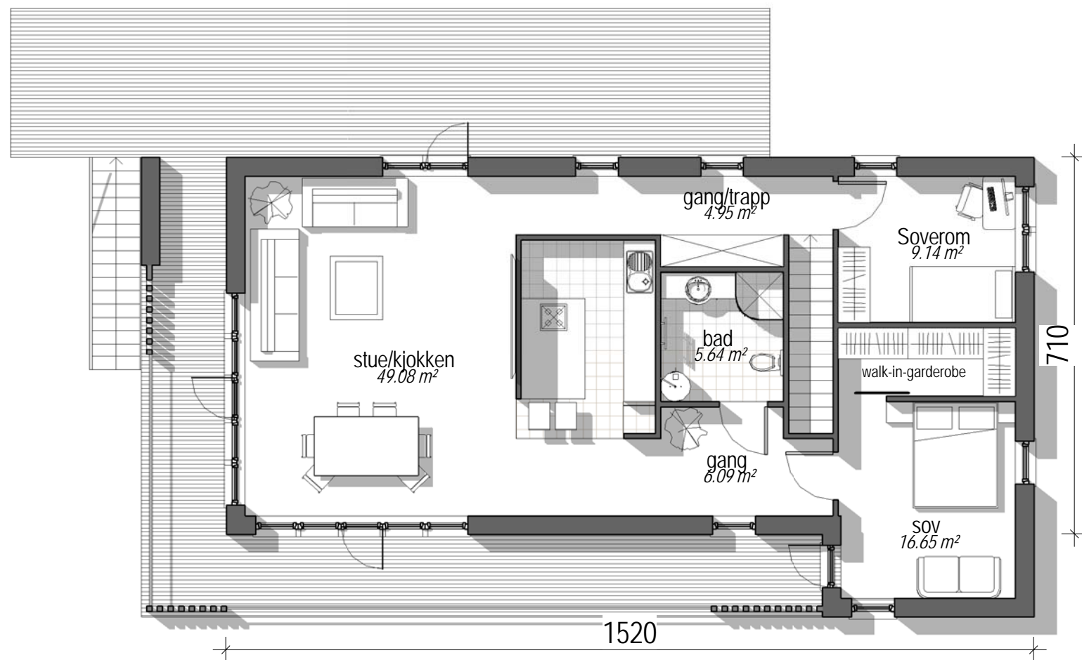
E2 - Plan andre etasje M 1 : 100
